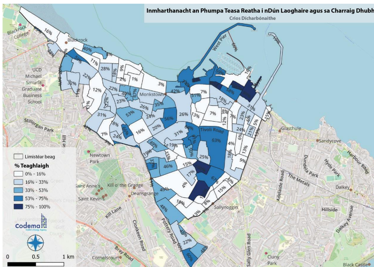
Figiúr 6.15 - Feiliúnacht do phumpaí teasa i ZD Dhún Laoghaire/na Carraige Duibhe
