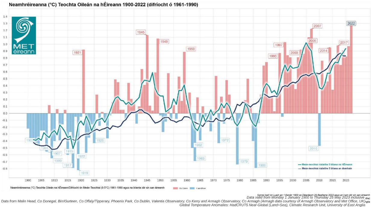
Fíor 1.1: Neamhréireanna (°C) Teochta Oileán na hÉireann 1900-2022 (difríocht ó 1961-1990) (Foinse: Met Éireann 2 )
